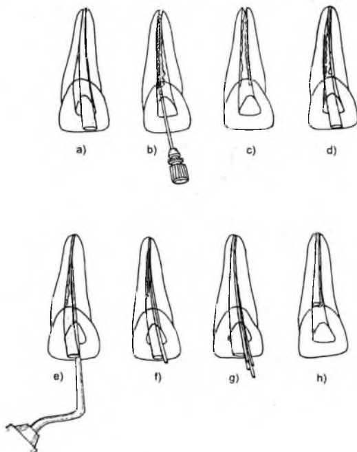
Hình 4.13. Kỹ thuật lèn ngang
